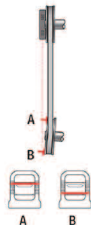
不对中
